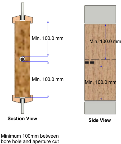
Optional Aperture Cut Section
