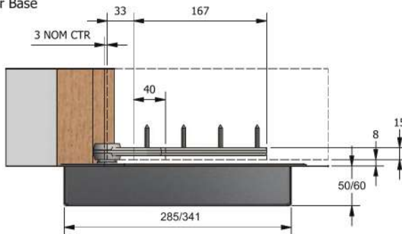
Door Base
