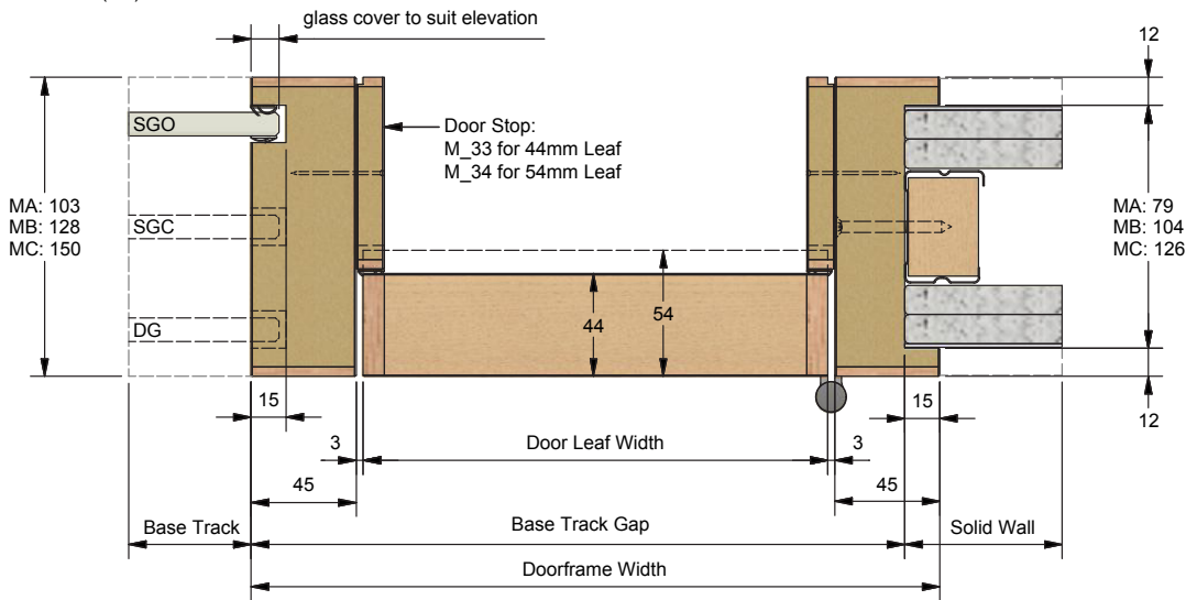
Door Jambs (1:3)
